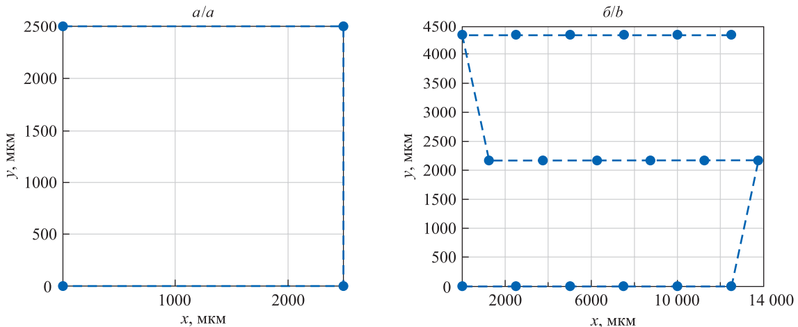
Рис. 4. Координаты экспонирования квадратной (а) и гексагональной (б) упаковки массива линз
