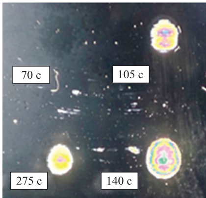
Рис. 5. Микрофотография ориентации ЖК в ячейке при разном времени экспонирования (плоскость ячейки расположена под углом 45^\circ в скрещенных поляризаторах)
