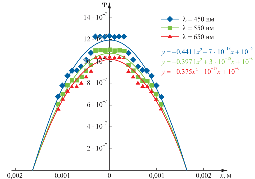
Рис. 10. Фазовый профиль ЖК-линзы
