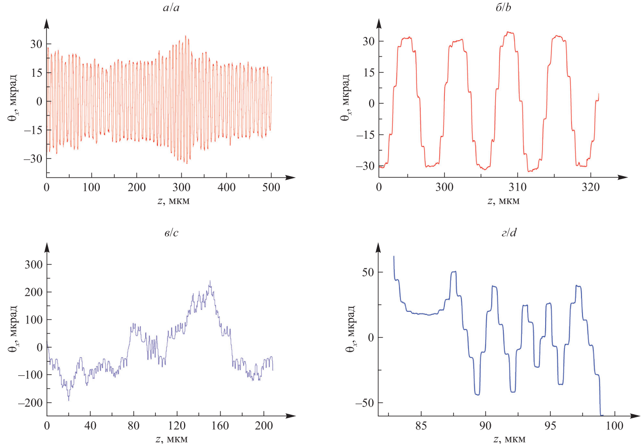
Рис. 2. Представленные в разных масштабах зависимости поперечной компоненты скорости позитрона ( a, б ) и электрона ( в, г ) с энергией 10 ГэВ от продольной координаты
