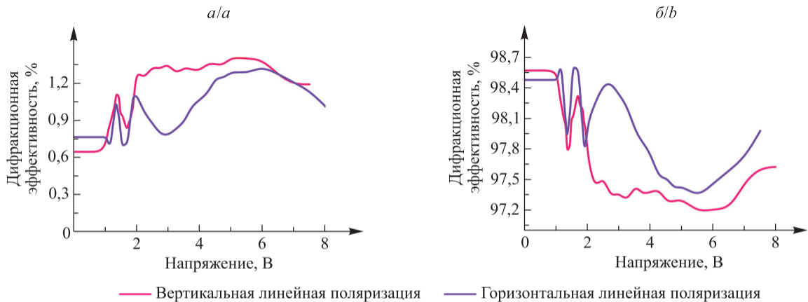
Рис. 4. Зависимости дифракционной эффективности от управляющего напряжения при линейной (вертикальной и горизонтальной) поляризации считывающего излучения: a – для порядка дифракции m = -1 ; б – для порядка дифракции m = 0
