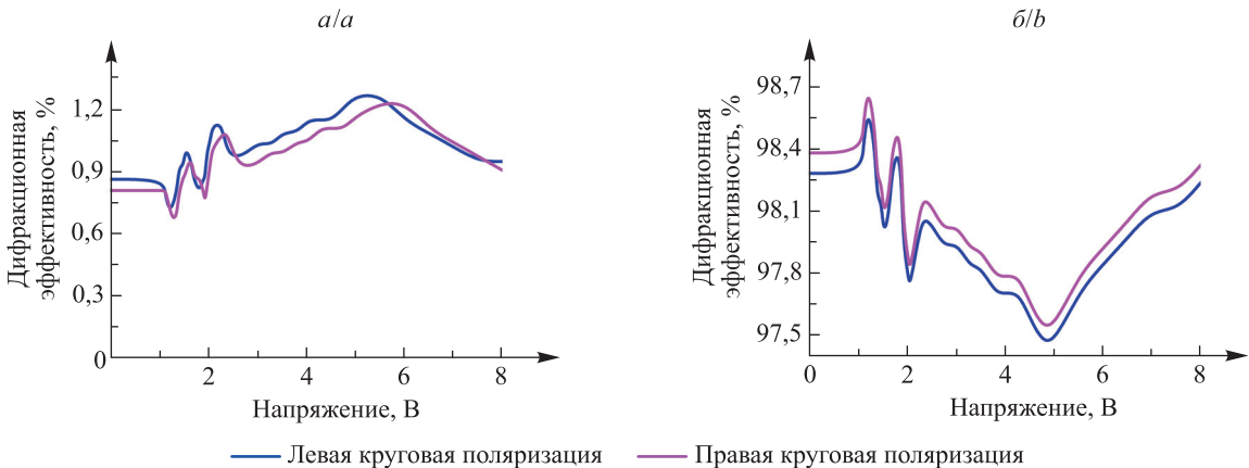
Рис. 5. Зависимости дифракционной эффективности от управляющего напряжения при круговой (левой и правой) поляризации считывающего излучения: a – для порядка дифракции m = -1 ; б – для порядка дифракции m = 0
