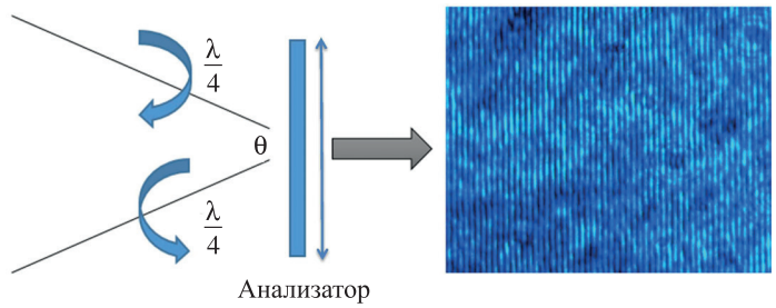
Рис. 6. Схемы сложения ортогональных поляризованных лазерных пучков и соответствующие микрофотографии результирующего светового поля: a – без использования анализатора; b – с использованием анализатора
