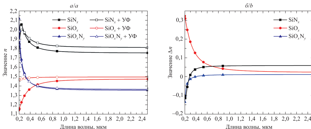
Рис. 2. Дисперсия показателя преломления (а) и разность спектров (б) образцов \text{SiN}_x , \text{SiO}_x , \text{SiO}_x\text{N}_y до и после УФ-воздействия
