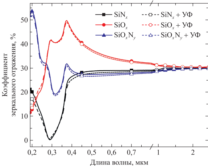
Рис. 1. Спектры зеркального отражения образцов \text{SiN}_x , \text{SiO}_x , \text{SiO}_x\text{N}_y до и после УФ-воздействия
