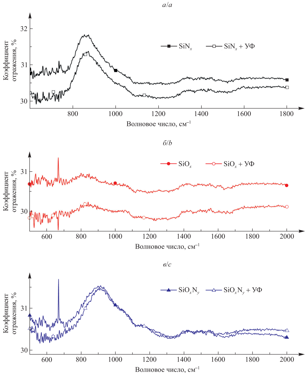
Рис. 3. Спектры ИК-отражения образцов \text{SiN}_x (а), \text{SiO}_x (б), \text{SiO}_x\text{N}_y (в) до и после УФ-воздействия
