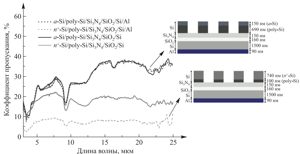
Рис. 3. Экспериментальные спектры пропускания структур \text{Si/Si}_3\text{N}_4\text{/SiO}_2\text{/Si} и \text{Si/Si}_3\text{N}_4\text{/SiO}_2\text{/Si/Al} до и после термического отжига
