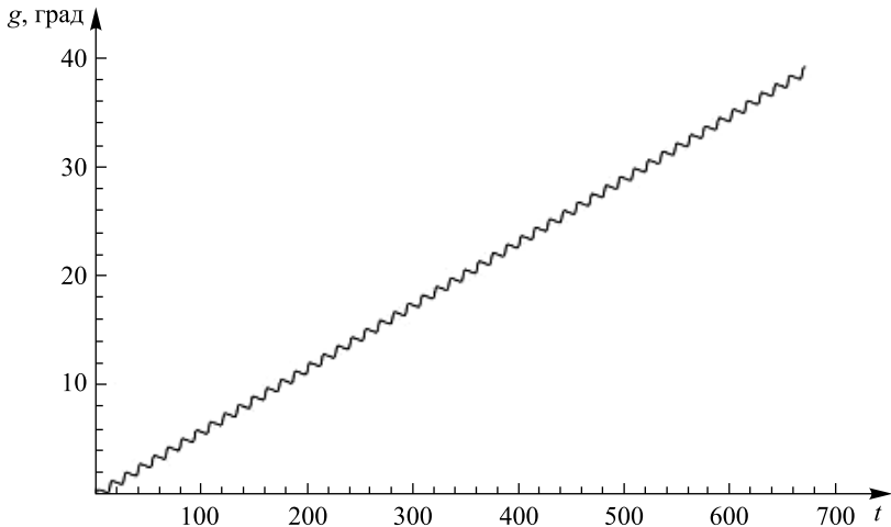
Рис. 3. Зависимость аргумента перицентра орбиты от времени Fig. 3. Time dependence of the argument of the periastron of the orbit
