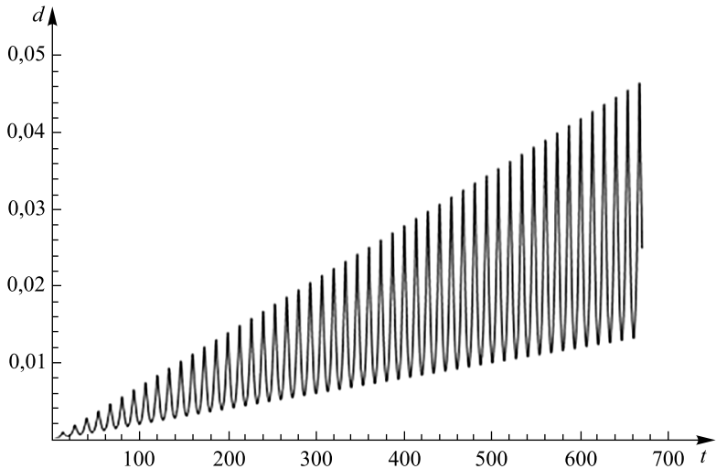
Рис. 4. Погрешность определения положения частицы (см. формулу (44))
