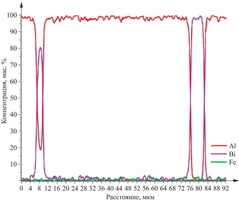
Рис. 2. Распределение элементов вдоль линии сканирования электронного луча на поверхности сплава Al – 1,3 мас. % Bi
