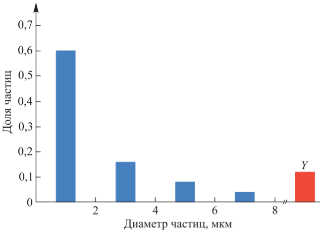
Рис. 3. Распределение частиц висмута сплава Al – 2,6 мас. % Bi по размерным группам
