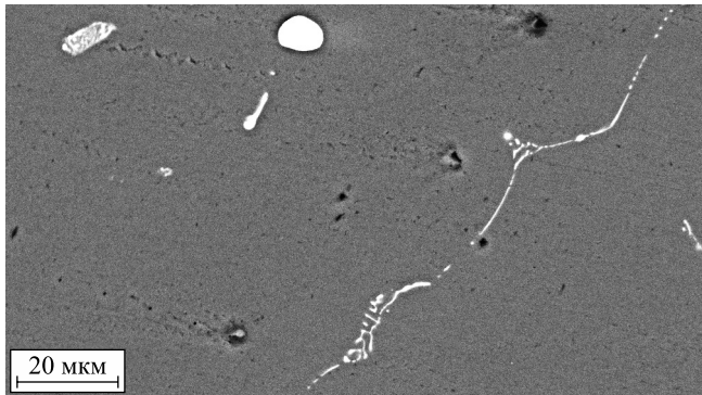
Рис. 4. Скопления выделений фаз в сплаве Al – 2,6 мас. % Bi
