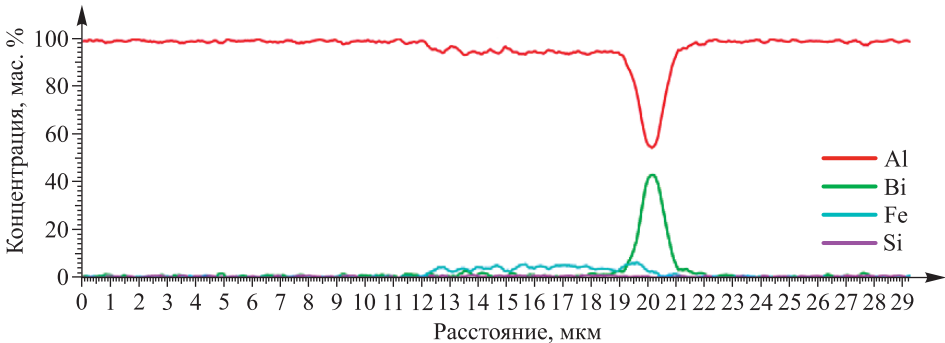
Рис. 5. Распределение элементов на участке, содержащем алюминий, висмут, железо и кремний, в сплаве Al – 2,6 мас. % Bi
