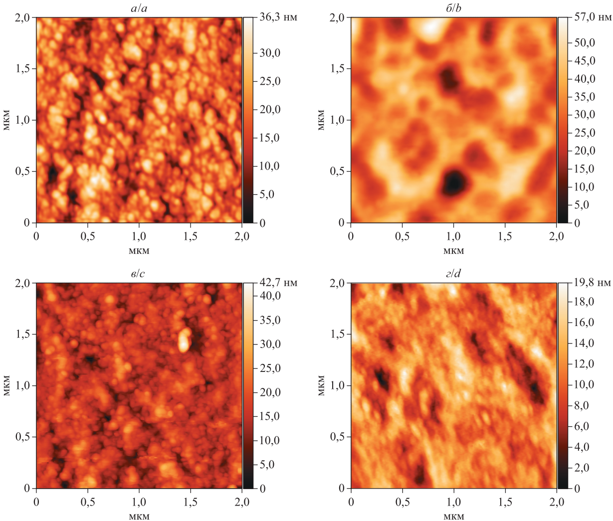
Рис. 5. АСМ-фотографии поверхности образцов покрытия TiAlCuN: a – образец 3N1; б – образец 3N2; в – образец 4N1; г – образец 4N2
