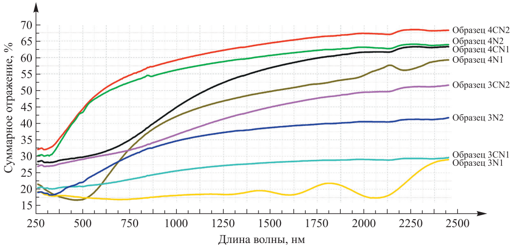
Рис. 6. Спектры суммарного отражения различных образцов покрытий TiAlCuN и TiAlCuCN Fig. 6. Total reflection spectra of various samples of TiAlCuN and TiAlCuCN coatings
