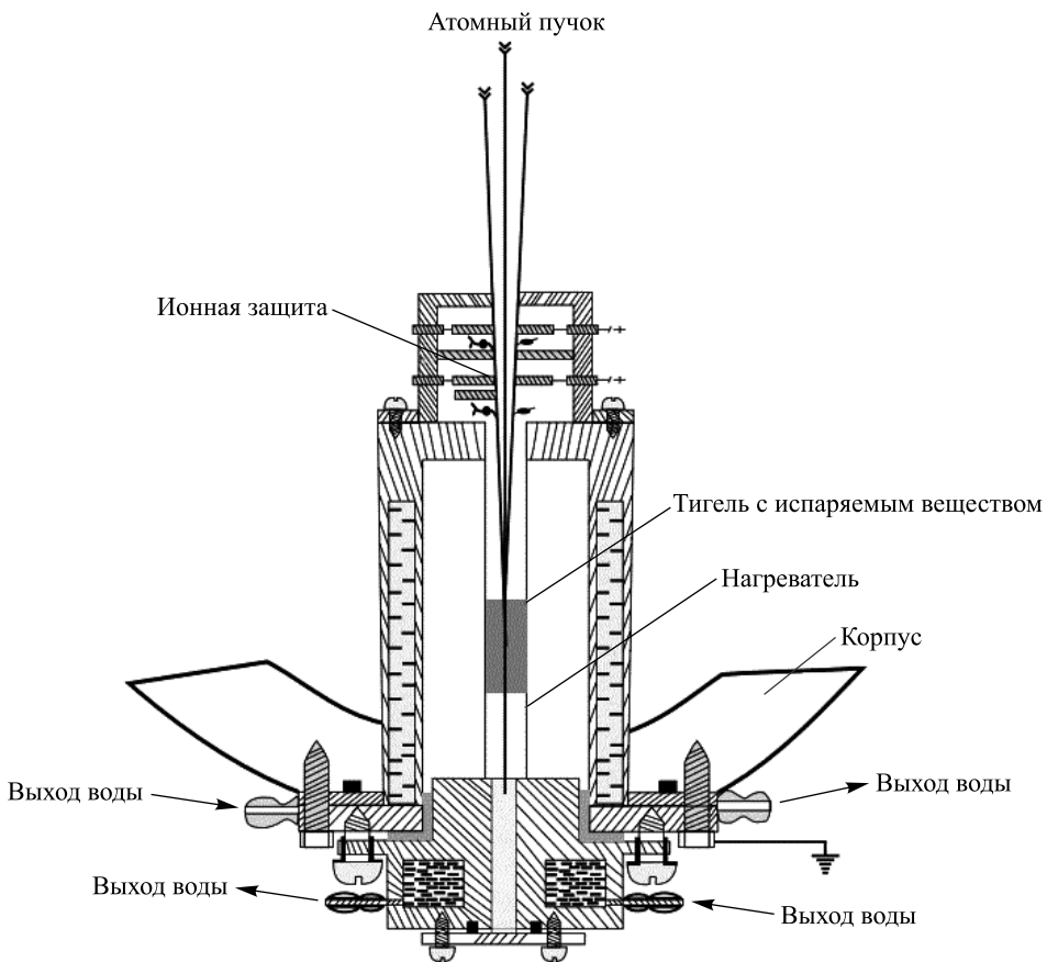
Рис. 3. Схема высокотемпературного источника нейтральных атомов
