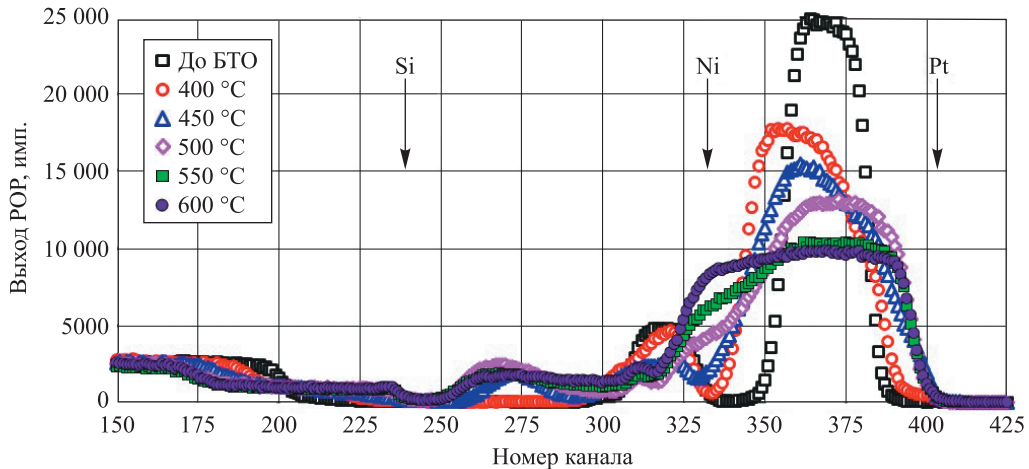
Рис. 2. Спектры POP, полученные от структуры Ni – V/Pt/Si с толщиной слоя сплава Ni – V 40 нм до БТО и после БТО при различных температурах
