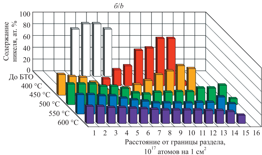
Рис. 3. Распределение концентраций атомов платины (а) и никеля (б) по толщине в структуре Ni – V/Pt/Si до БТО и после БТО при различных температурах
