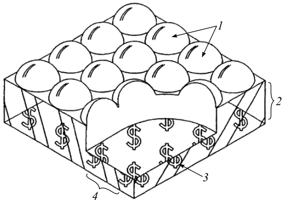
Рис. 1. Изометрический вид защитного устройства: 1 – микролинзы; 2 – толщина оптической прокладки; 3 – микроизображение; 4 – период микроизображения
