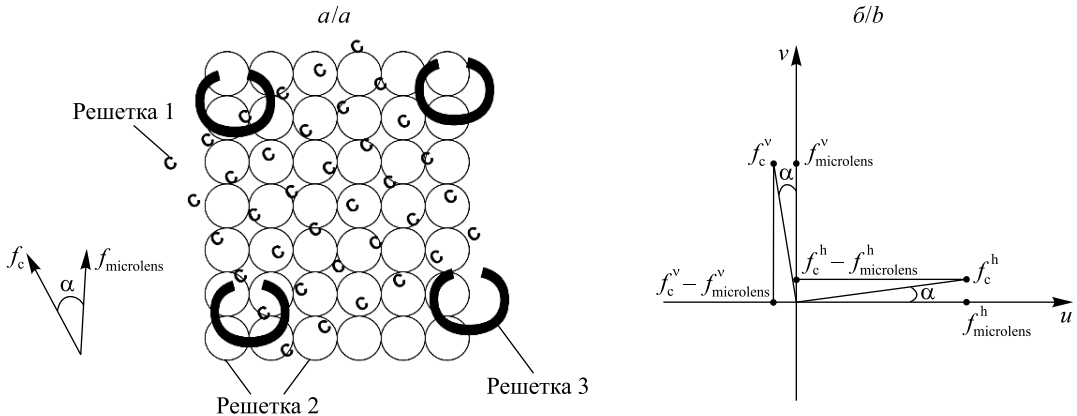
Рис. 7. Оптическая схема (а) и частотный спектр (б) защитного устройства с решеткой микроизображений «с», объединенной с решеткой микролинз
