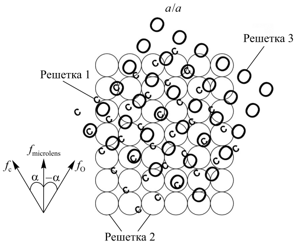
Рис. 8. Оптическая схема (а) и частотный спектр (б) защитного устройства с решетками микроизображений «с» и «О», объединенными с решеткой микролинз
