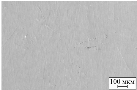
Рис. 1. РЭМ-изображения поверхности стали до обработки ЭП, полученные в режимах SE ( a ) и BSD ( б )
