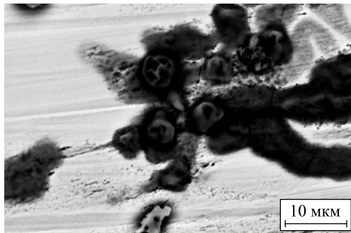
Рис. 2. РЭМ-изображения поверхности стали после обработки ЭП, полученные в режимах SE ( а, в ) и BSD ( б, г )
