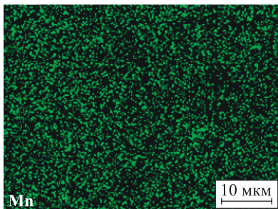
Рис. 3. Карты распределения химических элементов в стали после обработки импульсным ЭП
