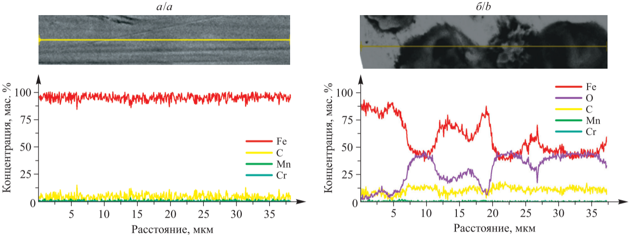
Рис. 4. Распределение химических элементов вдоль произвольной линии в приповерхностном слое исходного ( a ) и обработанного ЭП ( б ) образцов
