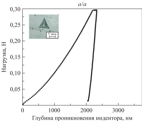
Рис. 7. Диаграммы инструментального индентирования «нагрузка – глубина проникновения индентора» исходного ( a ) и обработанного ЭП ( б ) образцов. На вставках приведены оптические снимки отпечатков индентора
