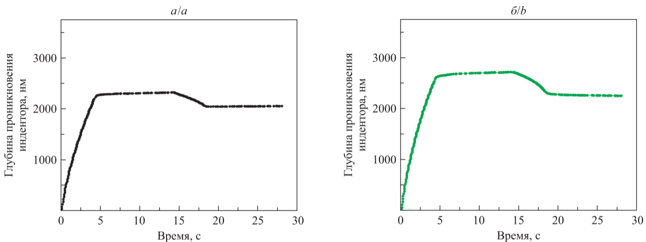
Рис. 8. Диаграммы инструментального индентирования «глубина проникновения индентора – время» исходного ( a ) и обработанного ЭП ( б ) образцов
