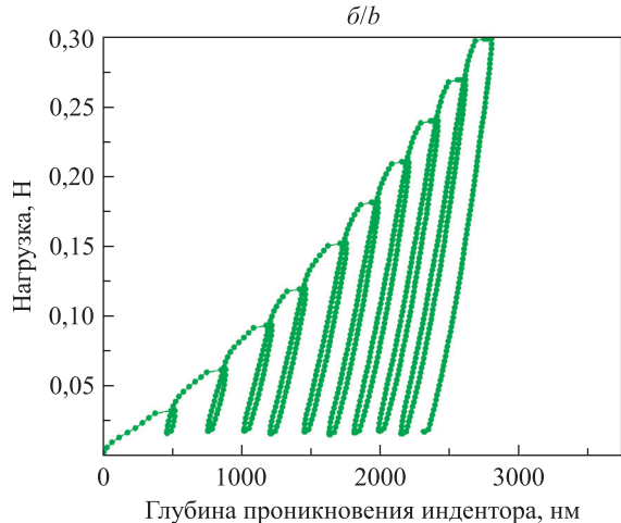
Рис. 9. Диаграммы инструментального индентирования «нагрузка – глубина проникновения индентора» исходного ( a ) и обработанного ЭП ( б ) образцов
