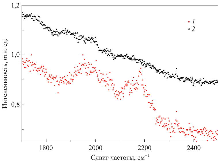
Рис. 3. Спектры КРС кремния (1) и твердого раствора \text{Si}_{1-x}\text{Ge}_x при x = 0,006 (2)
