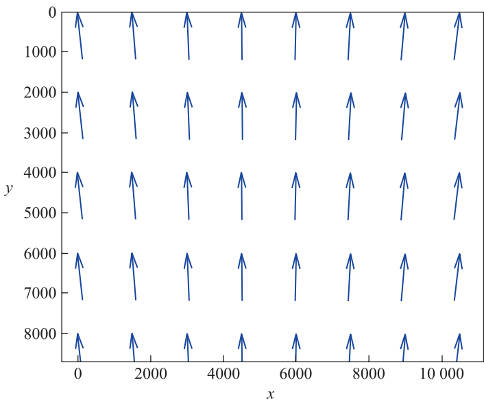
Рис. 8. Векторное поле «прообразов» и их призраков:
