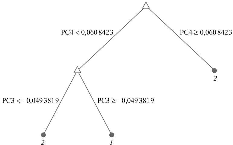
Рис. 6. Классификационное дерево для определения страны происхождения ромашки аптечной (1 – Россия; 2 – Беларусь) с выбором спектральных переменных
