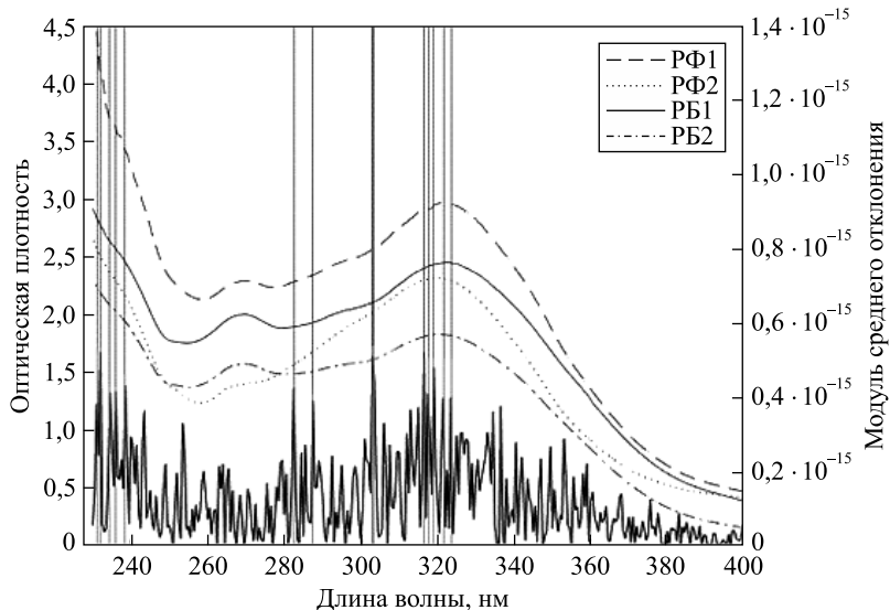
Рис. 8. Модуль среднего отклонения оптической плотности от усредненной величины (график черного цвета), спектры оптической плотности 70 % спиртовых настоек образцов ромашки аптечной и выбранные для проведения классификации производителя 14 спектральных переменных (вертикальные линии)
