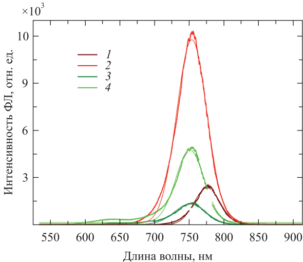
Рис. 1. Спектры ФЛ пленок \text{CH}_3\text{NH}_3\text{PbI}_3 (1, 2) и \text{CH}_3\text{NH}_3\text{Pb}(\text{I}_{0.57}\text{Cl}_{0.43})_3 (3, 4)
