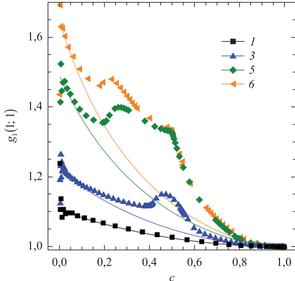
Рис. 7. Зависимость от концентрации корреляционных функций для ближайших соседей при \beta J = 0,10 (кривая 1); \beta J = 0,20 (3); \beta J = 0,40 (5) и \beta J = 0,50 (6).
