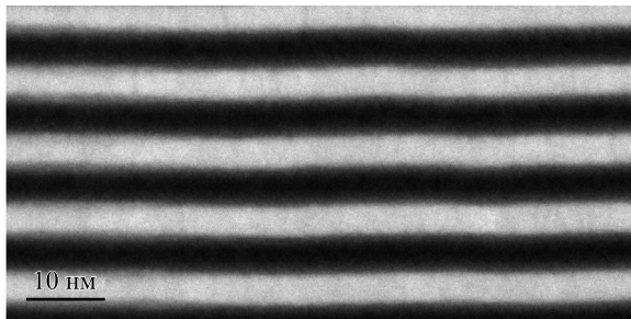
Рис. 2. HRTEM-изображения поперечных сечений многослойных покрытий \text{ZrN}/\text{SiN}_x : a – 2 нм/5 нм; б – 5 нм/5 нм
