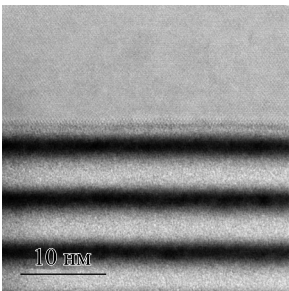
Рис. 2. HRTEM-изображения поперечных сечений многослойных покрытий \text{ZrN}/\text{SiN}_x : a – 2 нм/5 нм; б – 5 нм/5 нм
