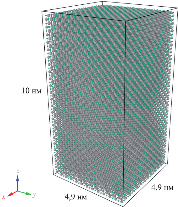
Рис. 1. Столбчатый TiN-нанокристалл высотой 10 нм
