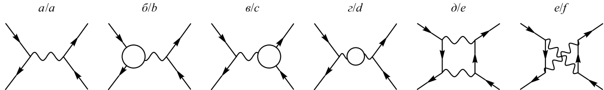
Рис. 1. Диаграммы Фейнмана для V -вклада в однопетлевом приближении: a – борновские амплитуды; б, в – вершинные диаграммы; г – собственно-энергетические диаграммы; д, е – диаграммы обмена двумя бозонами
