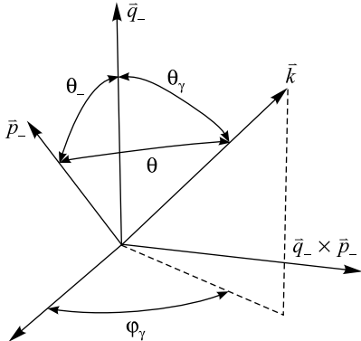
Рис. 3. Углы между векторами моментов импульса в с. ц. и.
