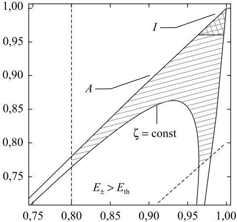
Рис. 4. Область интегрирования трехчастичного пространства
