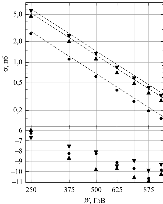
Рис. 5. Зависимость полного сечения от энергии столкновения в с. ц. и. при параметрах обрезания \zeta = 15^\circ , e = 0,5 .
