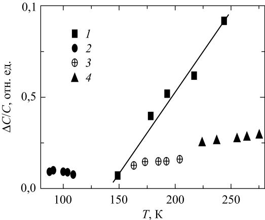
Рис. 2. Зависимости амплитуд пиков DLTS на рис. 1 (1–4) от температуры регистрации
