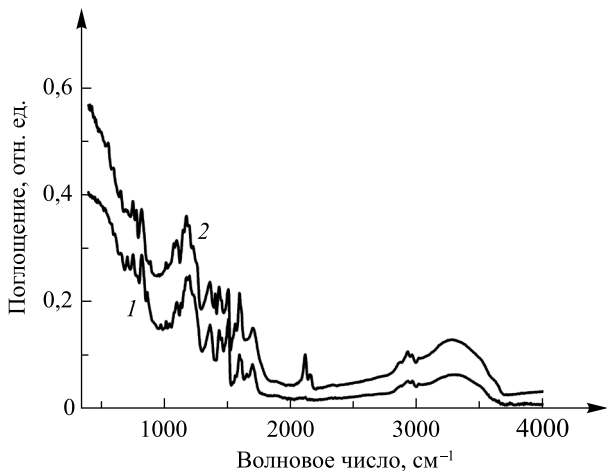
Рис. 2. Спектры НПВО пленок ФП9120 ( h = 2,5 мкм): 1 – исходных; 2 – имплантированных
