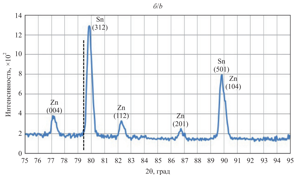
Рис. 1. Участки (а, б) рентгенограммы быстрозатвердевшей фольги
