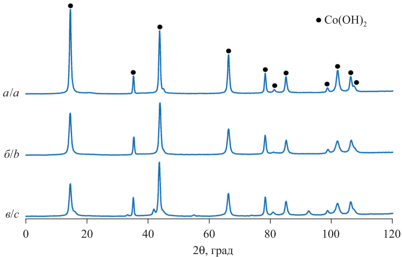
Рис. 2. Результаты РФА образцов, полученных при различных условиях: a – без ПАВ; b – с добавлением 0,1 % ЦПХ; c – с добавлением 0,1 % ДСН
