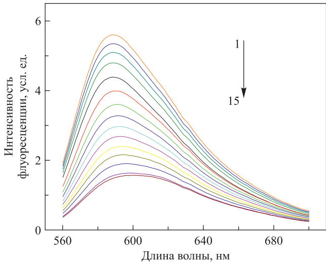
Рис. 3. Спектры флуоресценции Th-C11 в 97 % глицерине при температуре раствора 15–50 °С (сверху вниз, через 2,5 °С)
