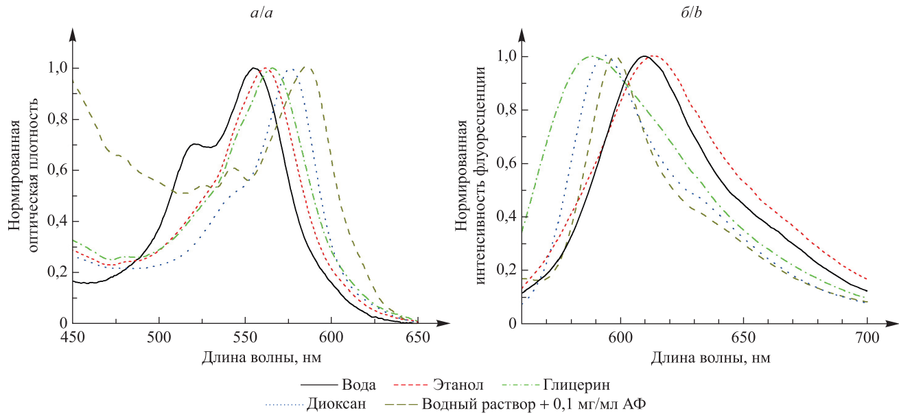
Рис. 6. Нормированные спектры поглощения (а) и флуоресценции (б) Th-C11 с концентрацией 5 \cdot 10^{-6} моль/л в различных растворителях
